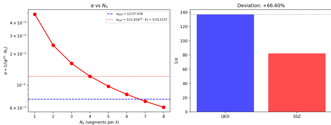
Abbildung 5.1: Abb. 5.1 — Geometrischer Ursprung von \alpha : \alpha = 1/(\varphi^{2\pi} \cdot N_0) als Funktion von N_0 (links) und Vergleich mit QED-Wert (rechts).
